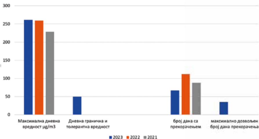
Мониторинг PM_{10} честица
