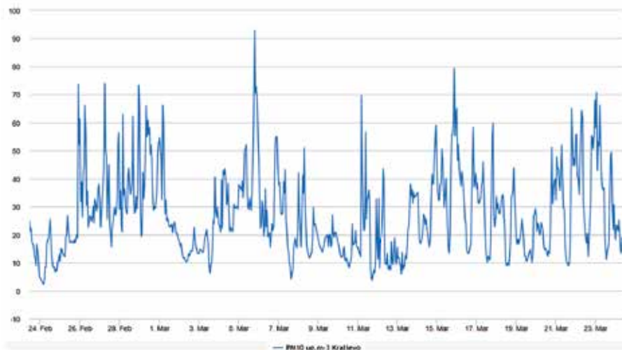
Сайни просеци PM_{10} честица у периоду од 24. 2. – 23. 3. 2024. године
